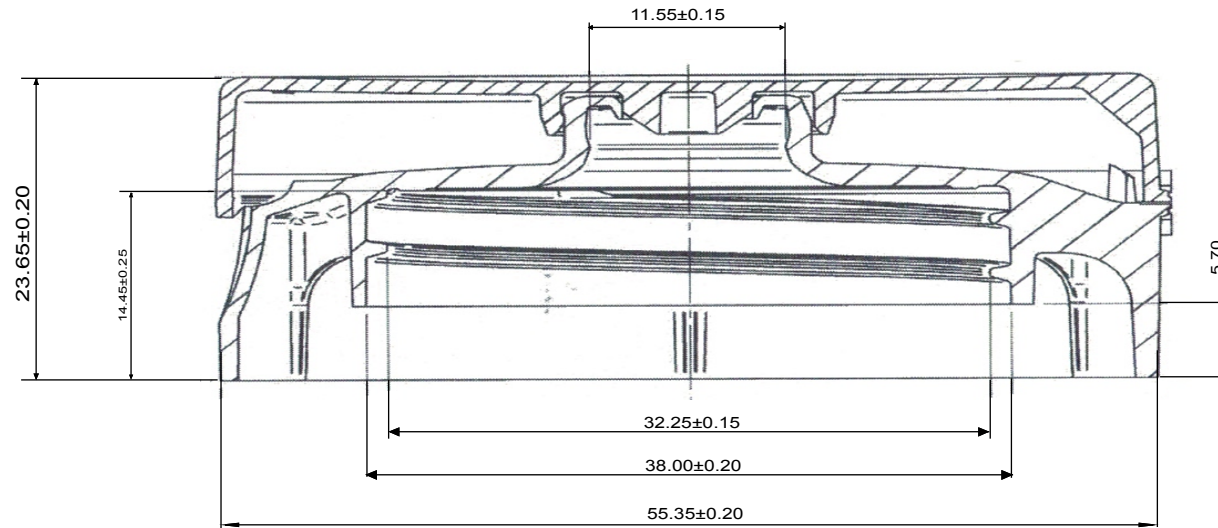
SECTION A-A 3:1
